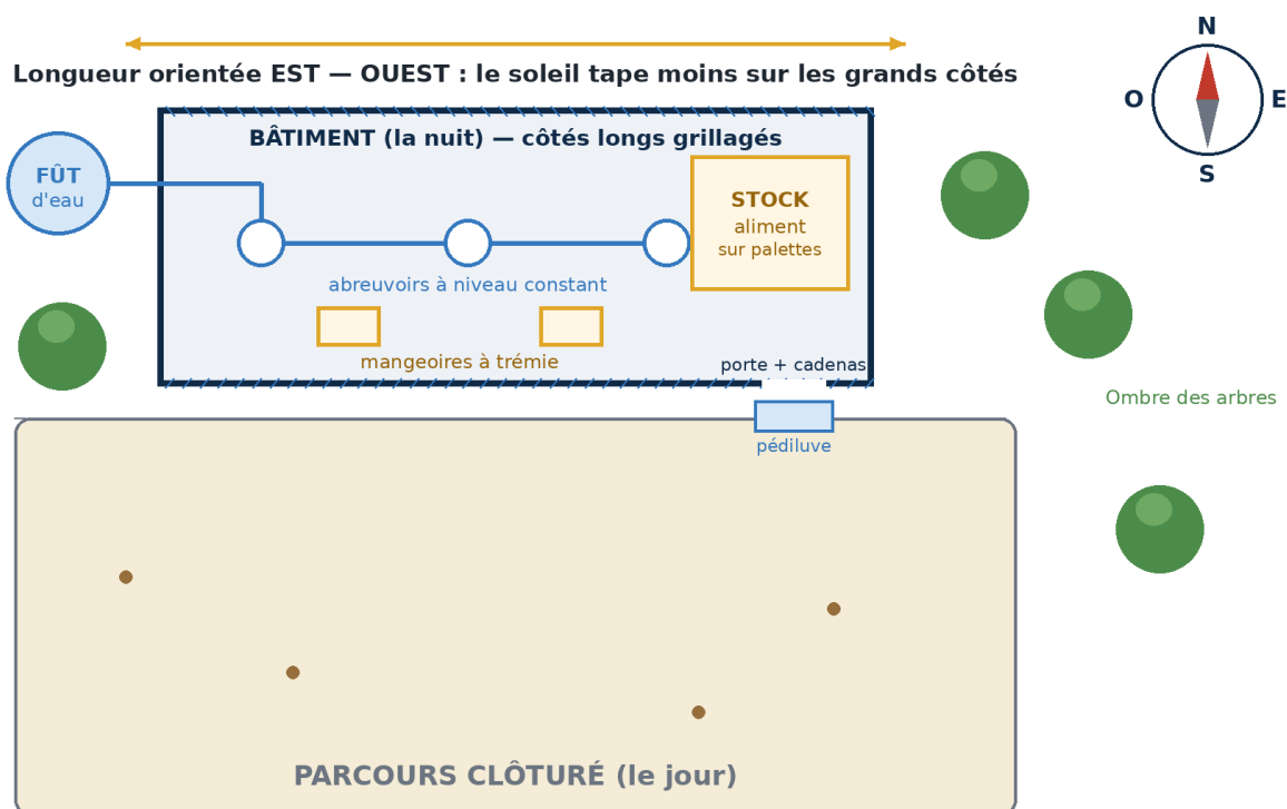
Schéma : un poulailler organisé pour limiter les interventions quotidiennes.
